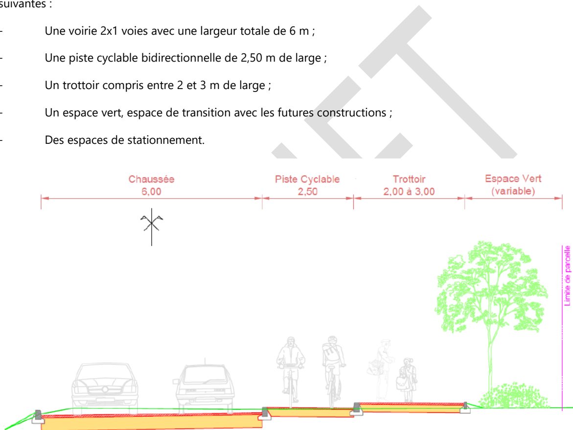
Figure 10 - Coupe de principe sud-nord du barreau Marcellin Allo (stade études préliminaires)
